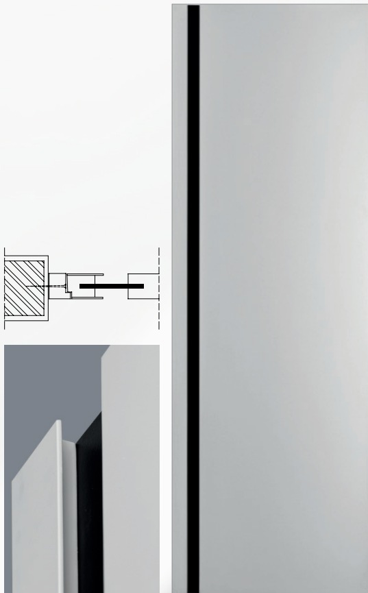
G 601 inzetstuk zwart deurdikte 48 mm
