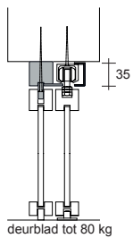
deurblad tot 80 kg
